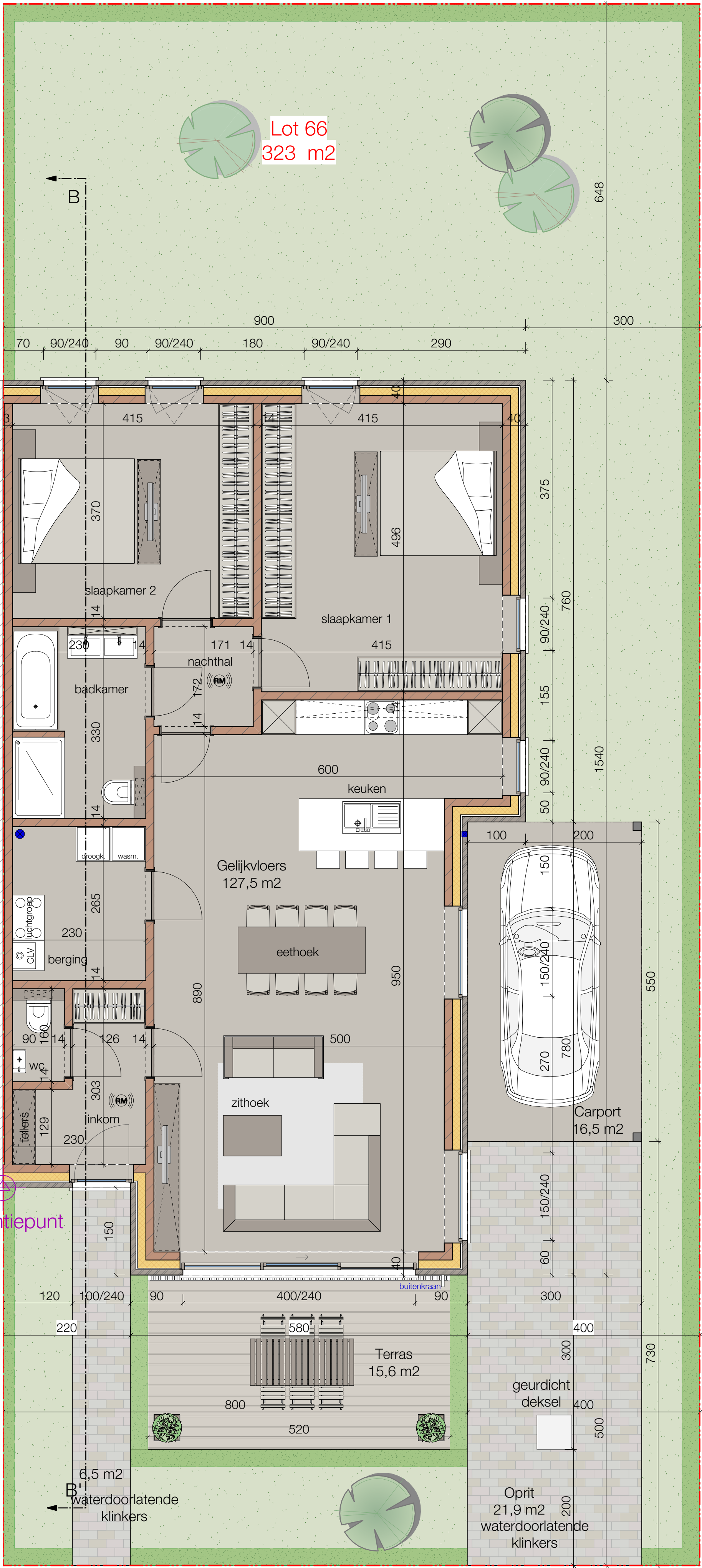
Gelijkvloers Schaal: 1:50
